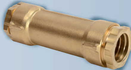
2 conexiones REXUO con cuerpo largo y pasante - Ø ext. de 20 a 63mm
