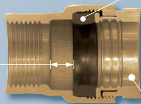
Sección de un SE14
